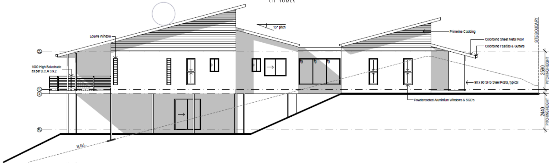
ELEVATION 4 - 1:100
