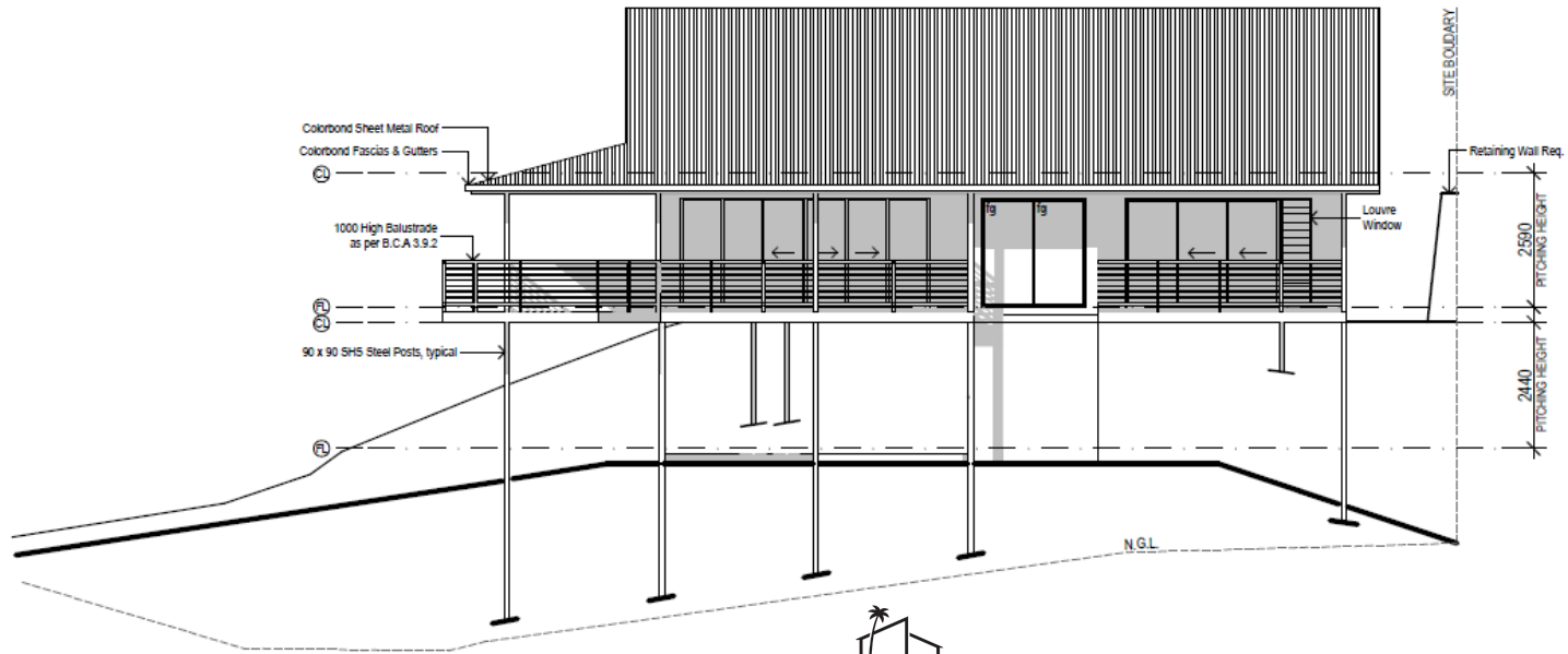
ELEVATION 3 - 1:100
