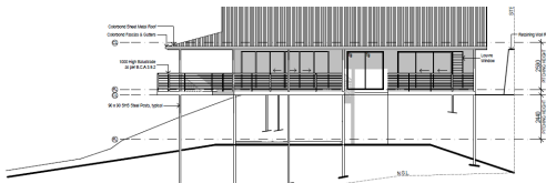
ELEVATION 3 - 1:100
