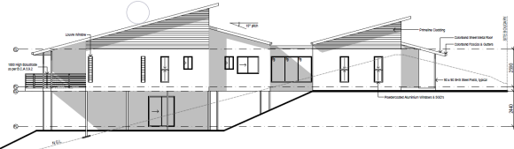
ELEVATION 3 - 1:100
